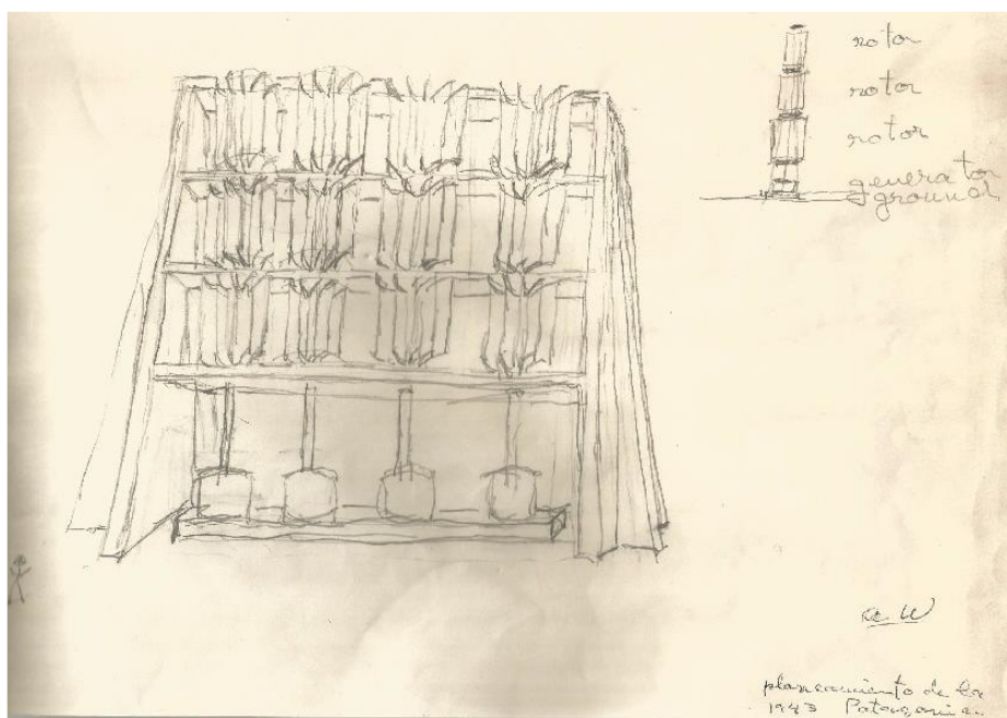
Fig. 26. Turbinas de eje vertical. Fuente: Archivo Amancio Williams
